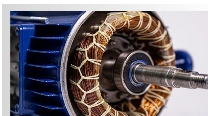
Infasurare stator din cupru
