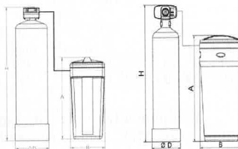
Dimensiunile echipamentelor SOFT SIMPLEX
