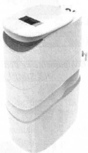
Vedere generala echipamentelor de dedurizare SOFT CAB LOTUS
