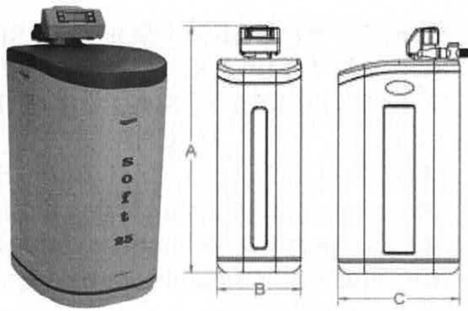
Dimensiunile echipamentelor SOFT CAB
